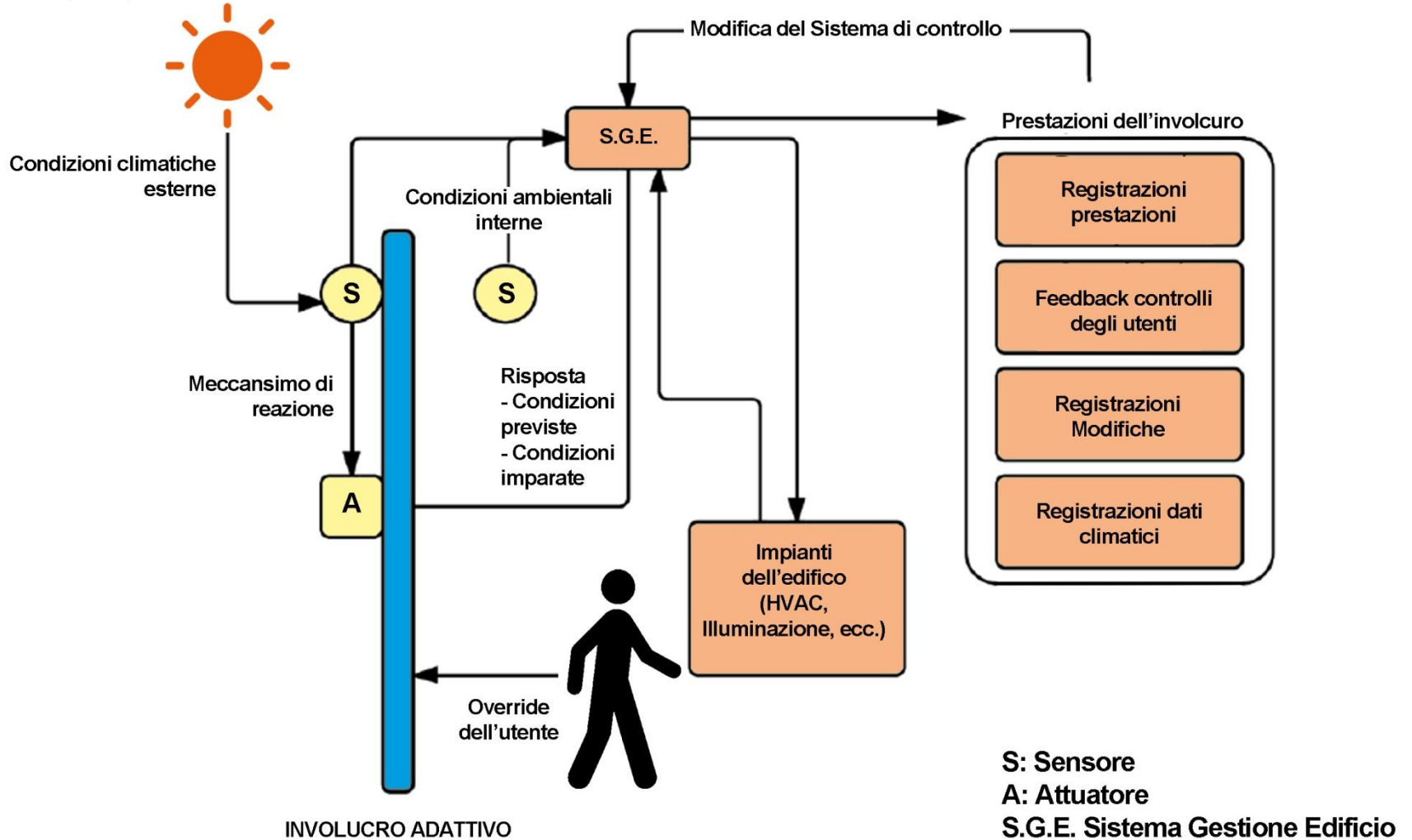
Schema di principio di funzionamento di un involucro adattivo
