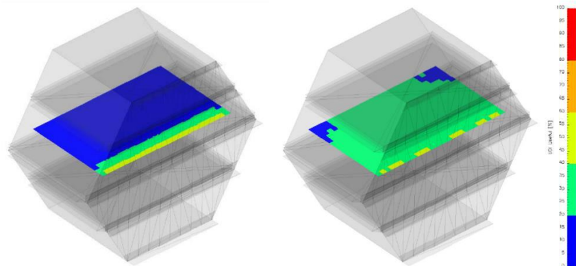
Confronto dei livelli di illuminazione naturale utili senza e con sistema di schermatura esterna
