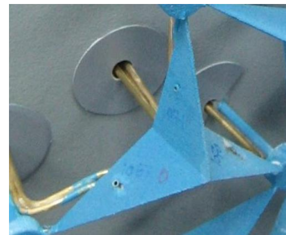
Particolare del sistema attuatore degli schermi triangolari
