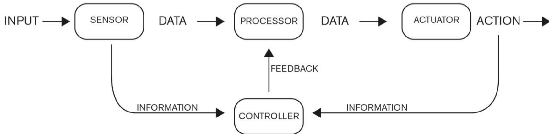
Schema di flusso di un sistema ciclico chiuso con unità di controllo
