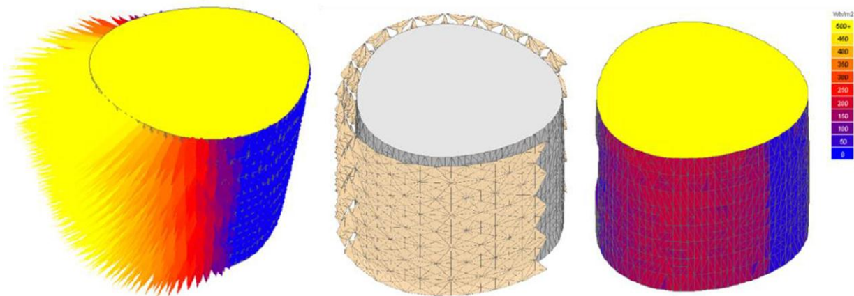
Analisi cumulativa della radiazione solare totale nel periodo estivo senza e con sistema di schermatura esterna
